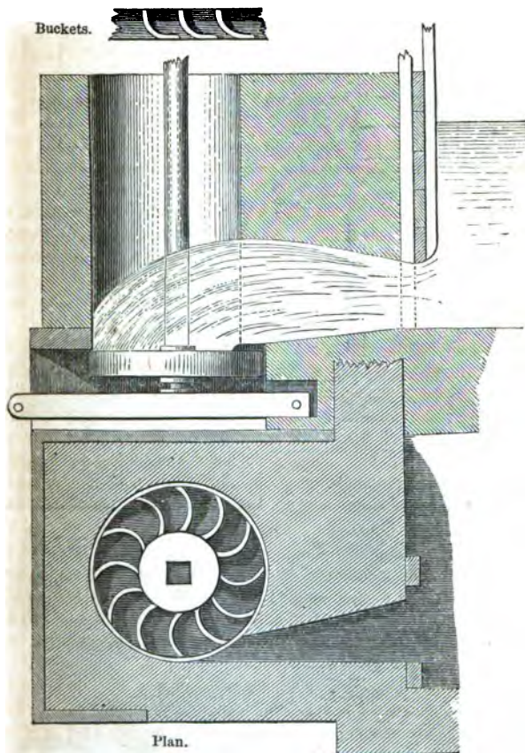
Fig. 8.—Roue à Cuves.
